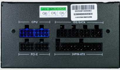
Entrada para os cabos
