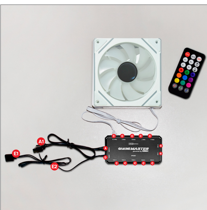
DIAGRAMA DE CONEXÕES
